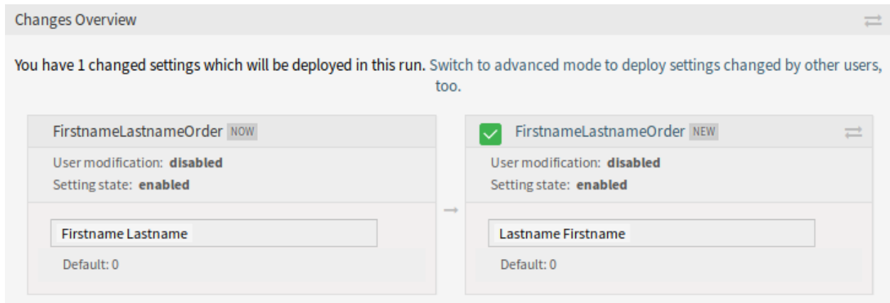
图 38: 系统配置 - 设置差异情况
