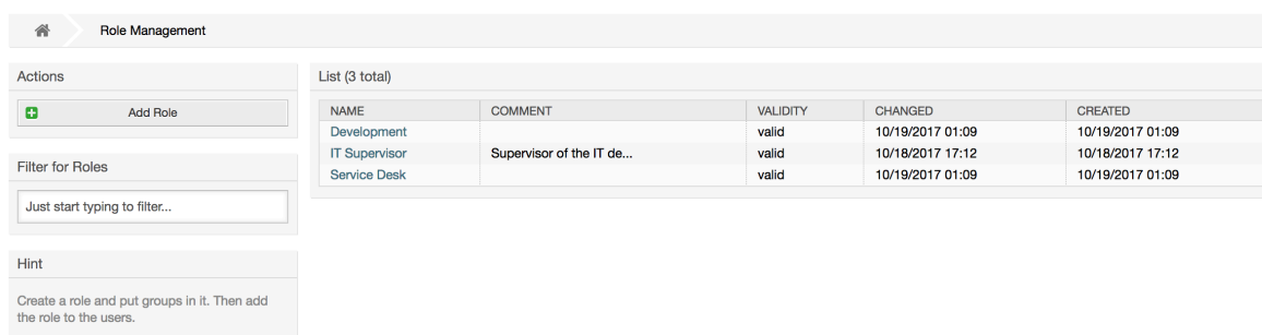
图 4.8. 角色管理
