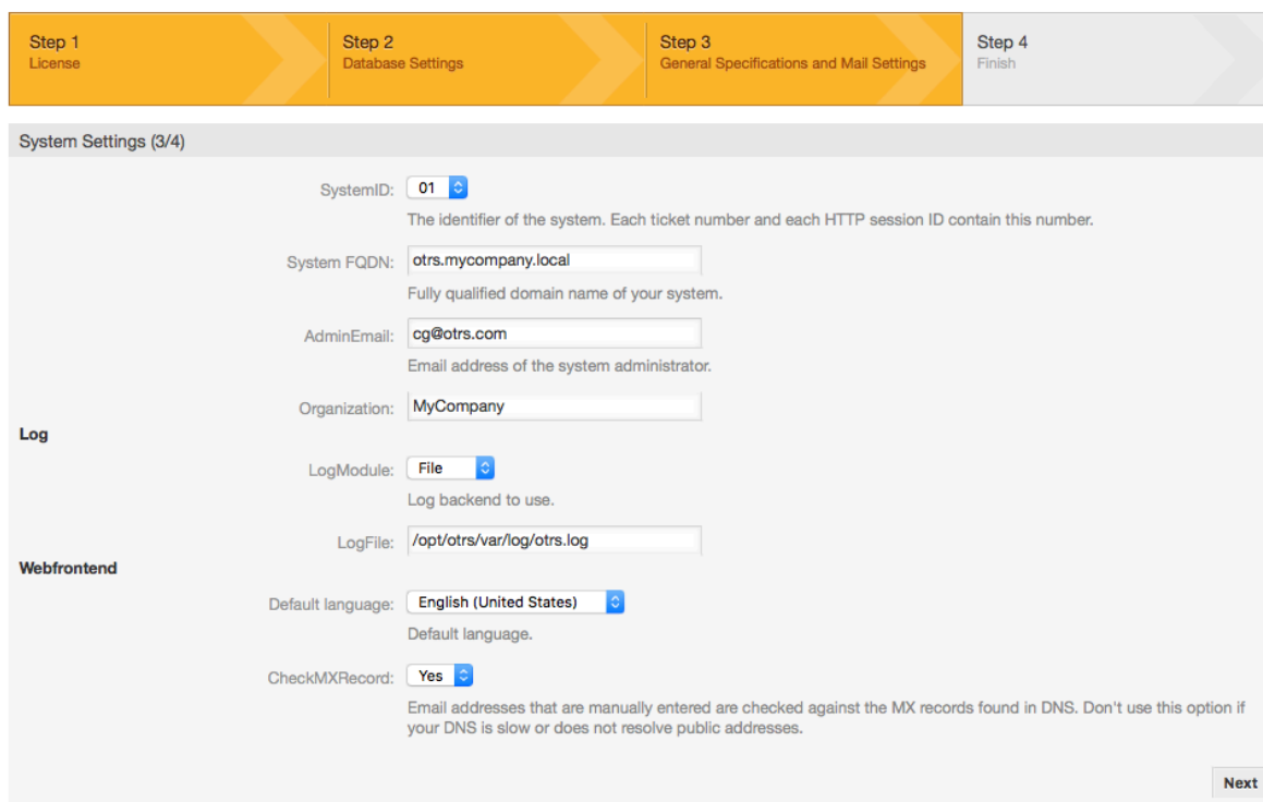
图 2.7. 系统设置
