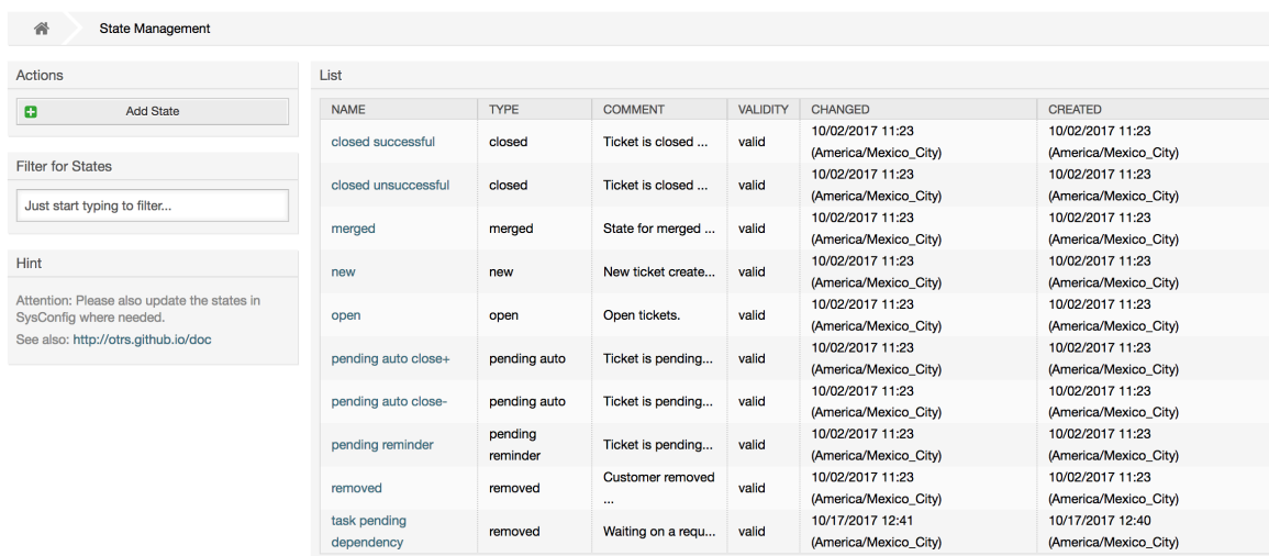
图 4.52. 状态管理
