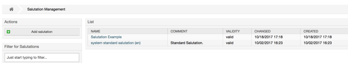
图 4.26. 问候语管理
