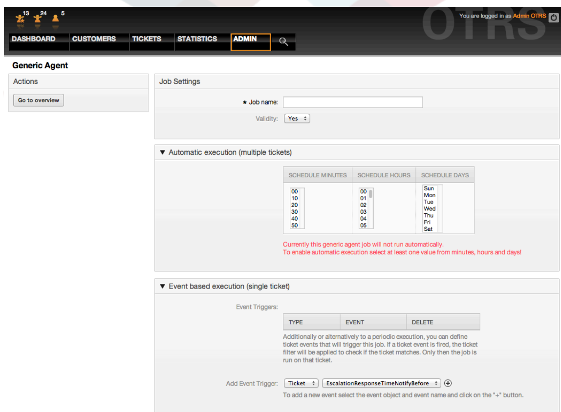
Рисунок: Создание заданий для GenericAgent.
